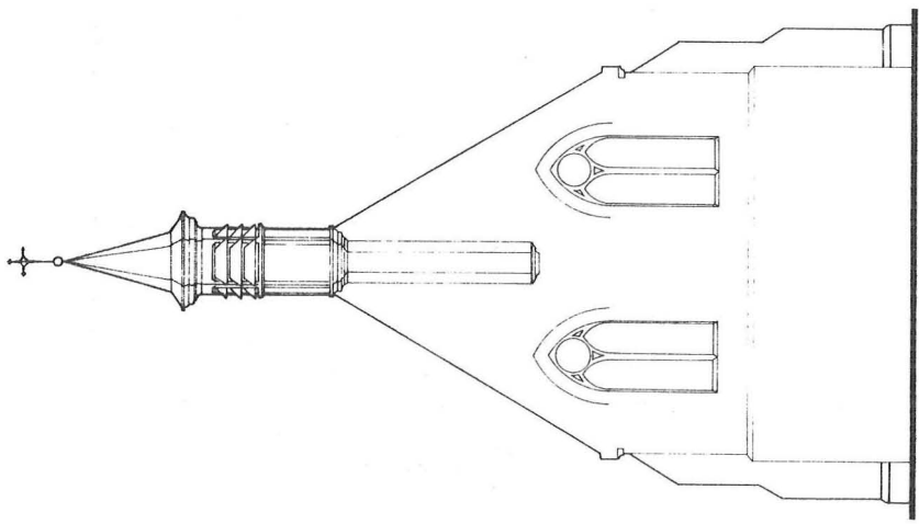
RECONSTRUCTIE VAN DE WESTGEVEL
