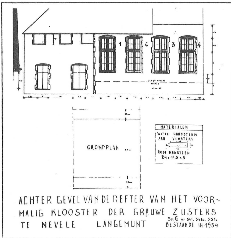
Plan van achtergevel van het klooster. Getekend door A. Janssens, konservator van het Rietgaverstedemuseum, vóór de gedeeltelijke afbraak. Archief Rietgaverstedemuseum, Nevele.
